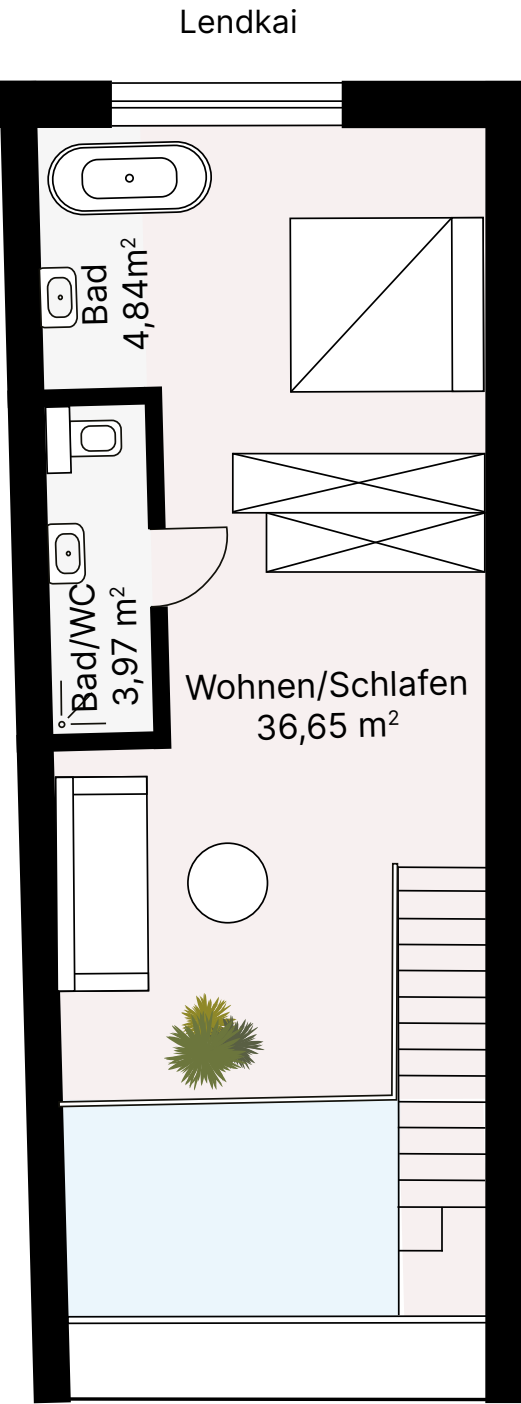
OG3 Innenhof
