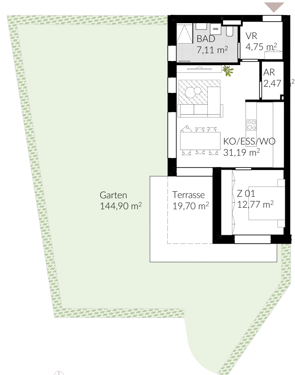
⌚ GRUNDRISS OBERGESCHOSS 1
